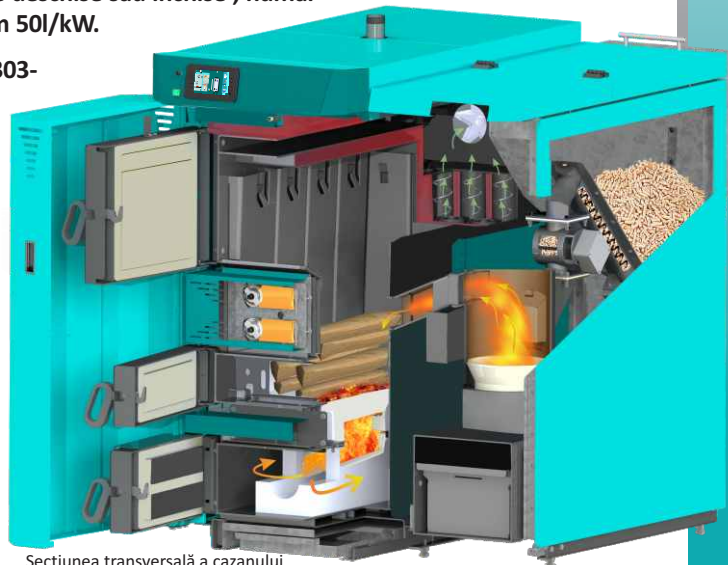
Secțiunea transversală a cazanului
